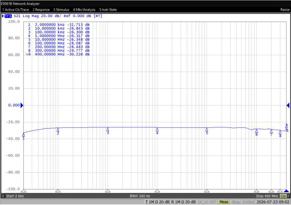
T-52 电流监测探头 s21 曲线
