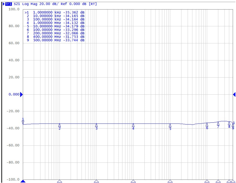
T-57 卡式电流监测探头 S21 曲线
