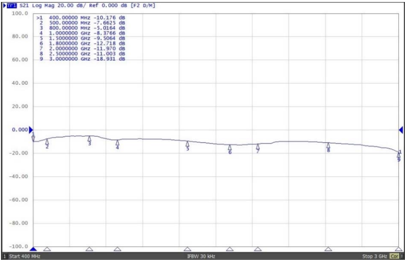
TWC 4013 管状波耦合器插入损耗（IL）测试曲线
