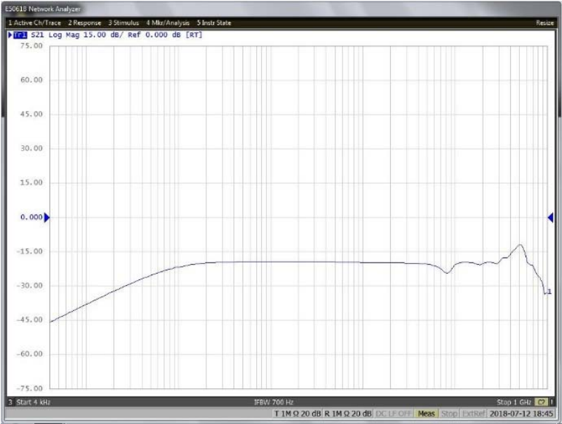
TWCM-500 卡式宽带电流监测钳 S21 曲线
