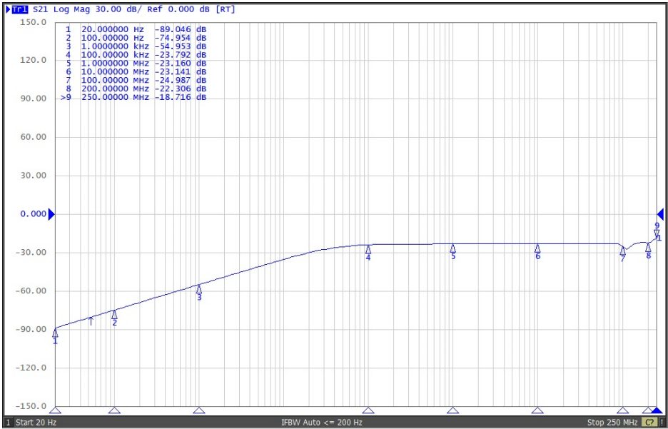
T-17A 卡式电流监测探头 s21 曲线
