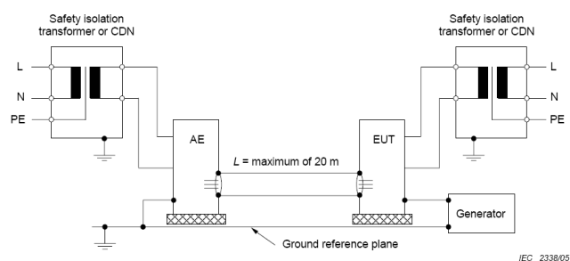
标准原理图 2 (屏蔽线一端接地)：
