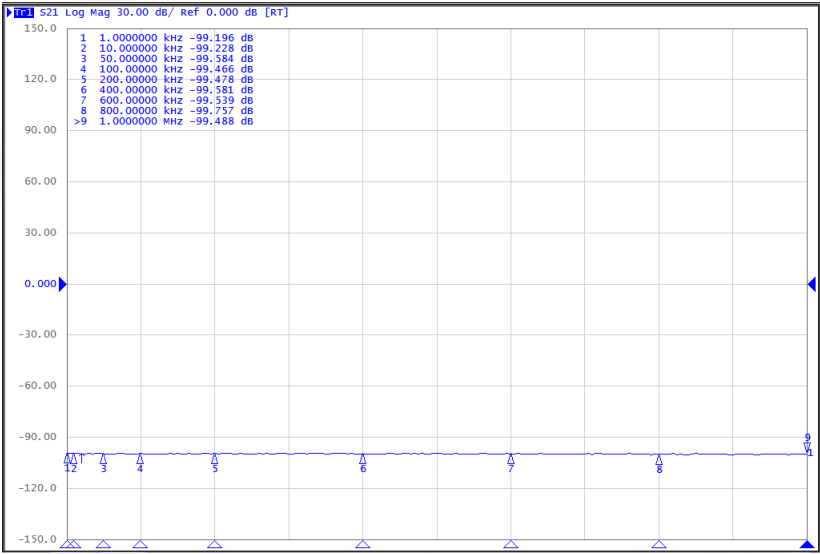
CCM 0301M宽带电流监测钳s21曲线（10 kHz ~ 1 MHz）
