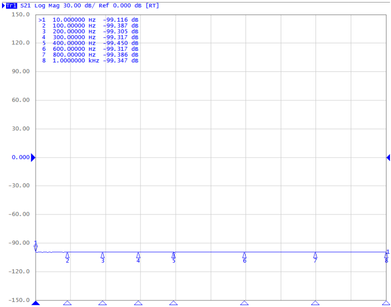
CCM 0301M宽带电流监测钳s21曲线（10 Hz ~ 1 kHz）
