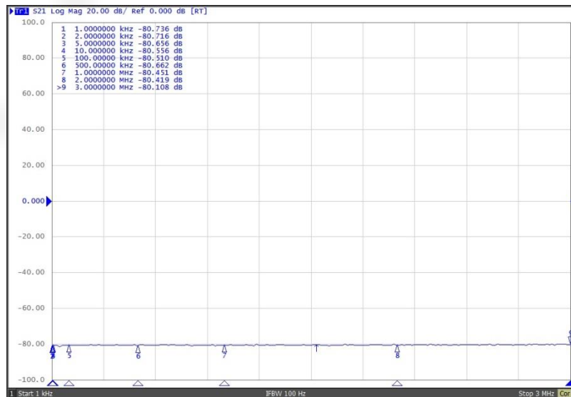
CCM 0203M卡式宽带电流监测钳s21曲线 (1 kHz ~ 3 MHz)
