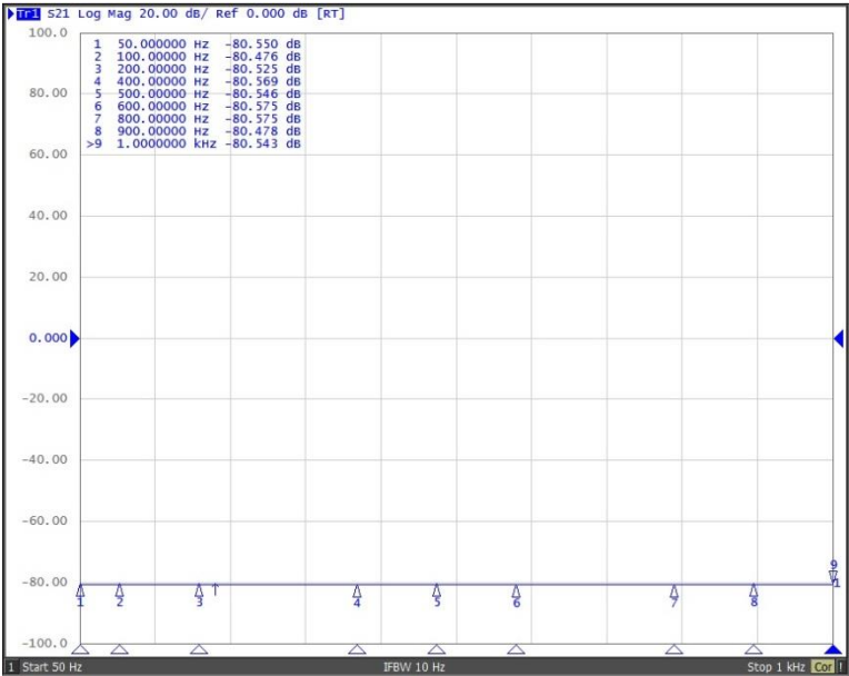
CCM 0203M卡式宽带电流监测钳s21曲线（50 Hz ~ 1 kHz）
